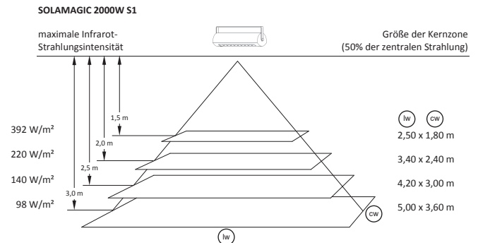
Strahlungspyramide SOLAMAGIC® S1 2000 W
